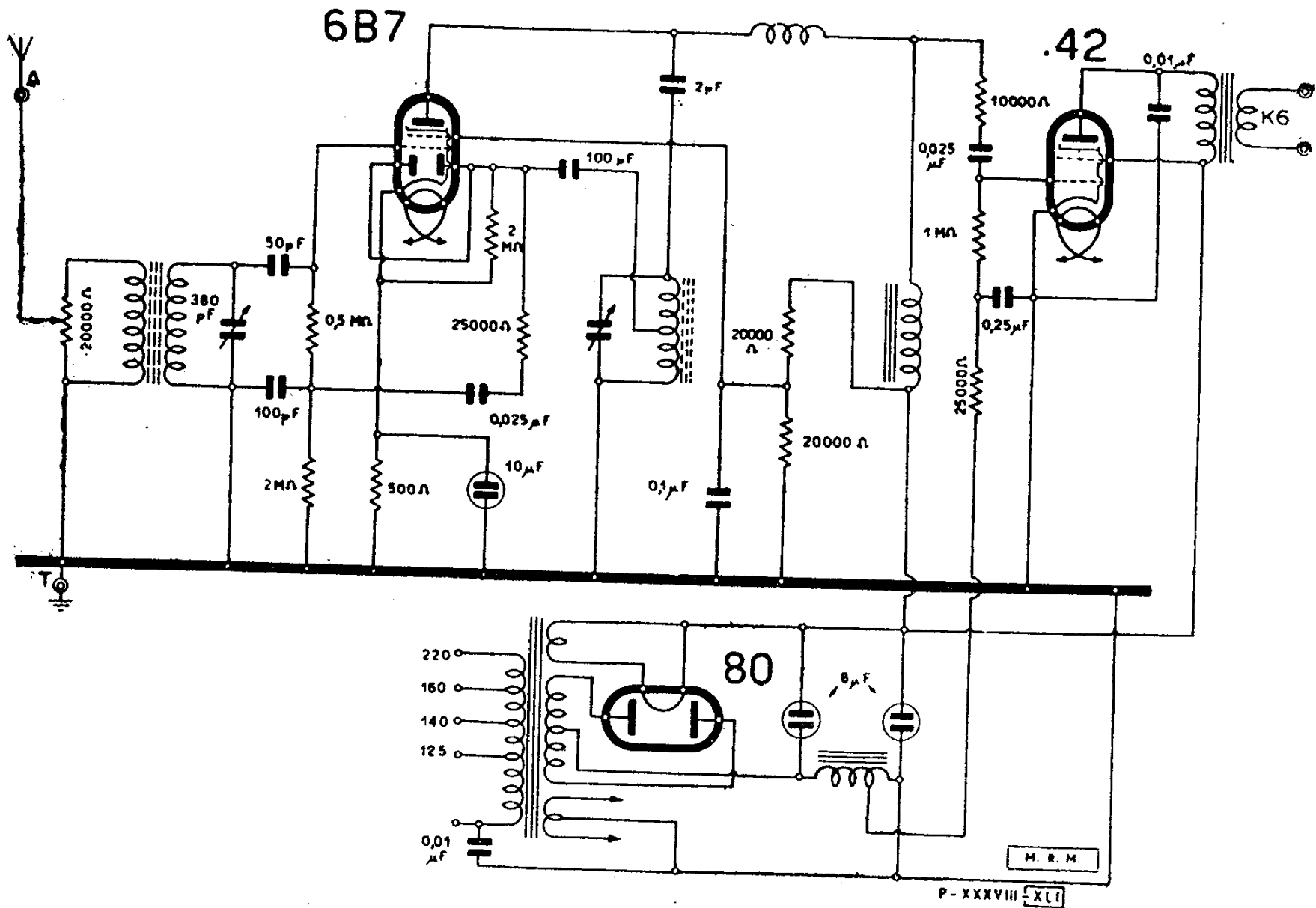
WATT RADIO - MOD. « BALILLA »
